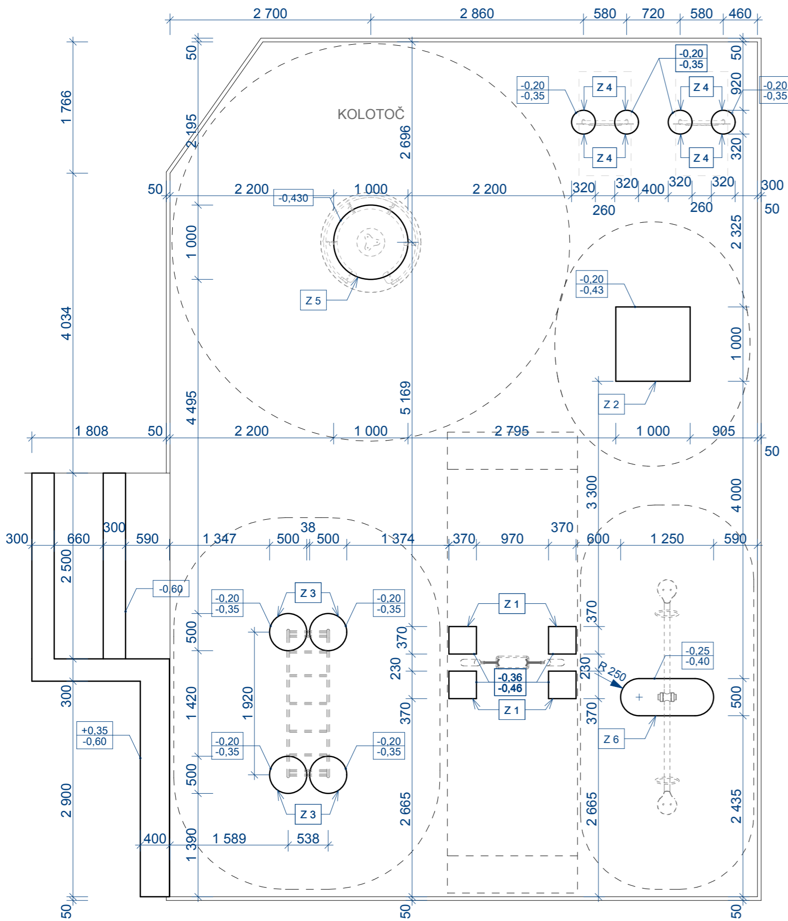
PÔDORYS ZÁKLADOV DETSKÉHO IHRISKA
