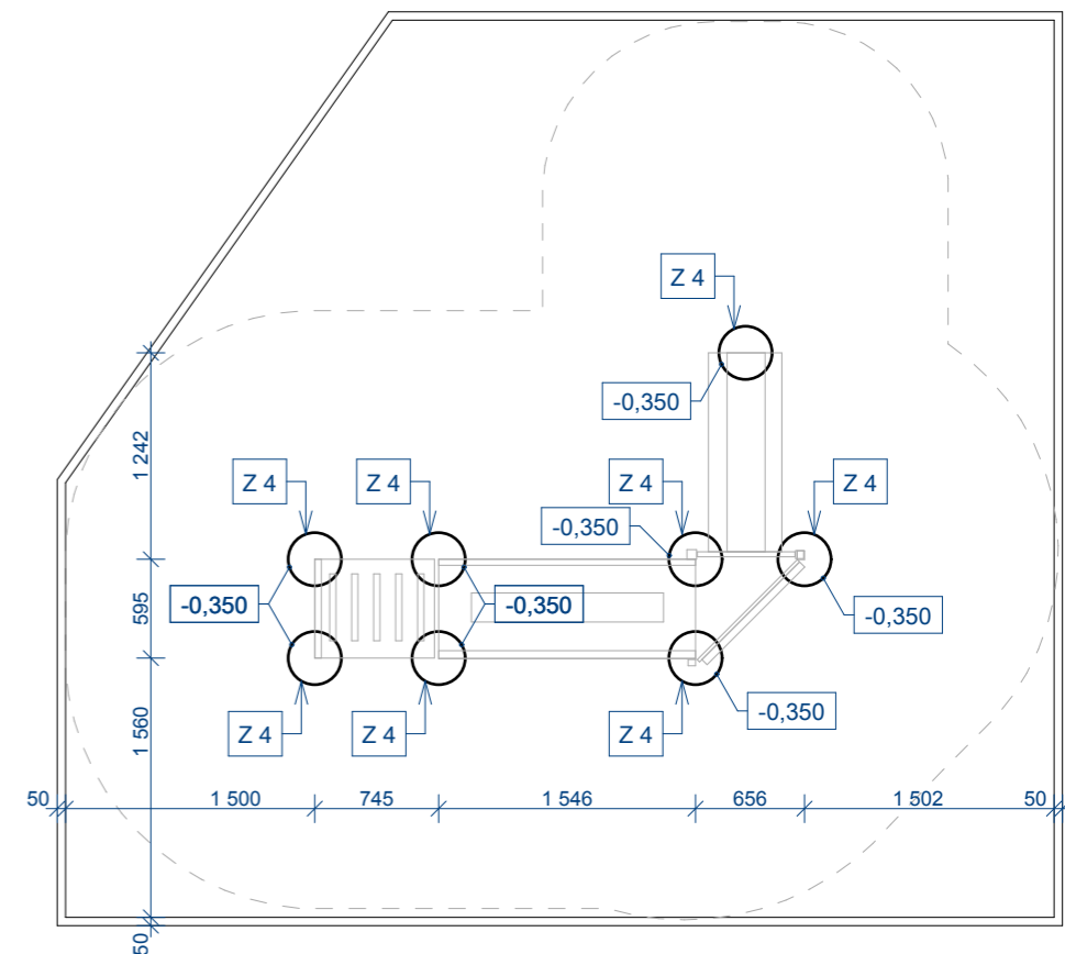
PÔDORYS ZÁKLADOV MALEJ LEZECKEJ ZOSTAVY
